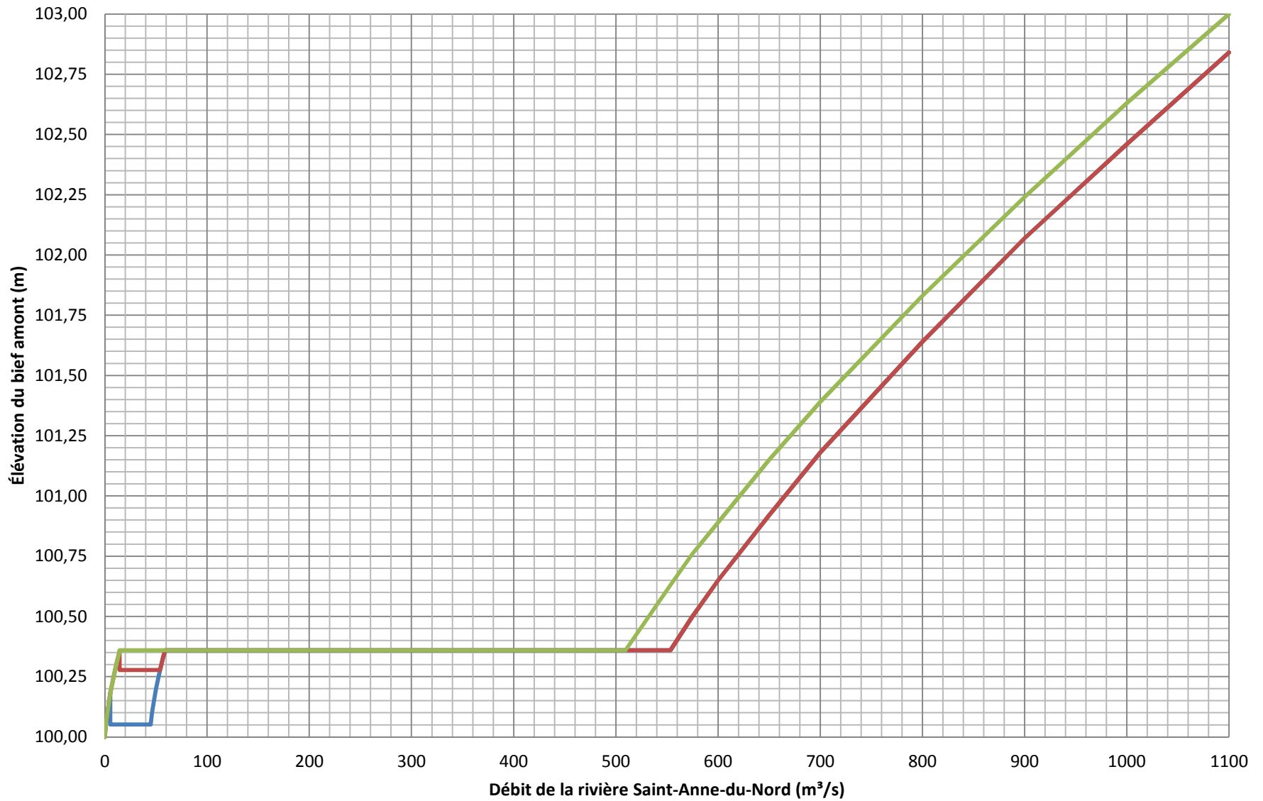
Figure A-1 : Courbe de tarage du bief amont (1/2)
